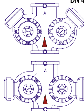
DN 40-50-65-80
